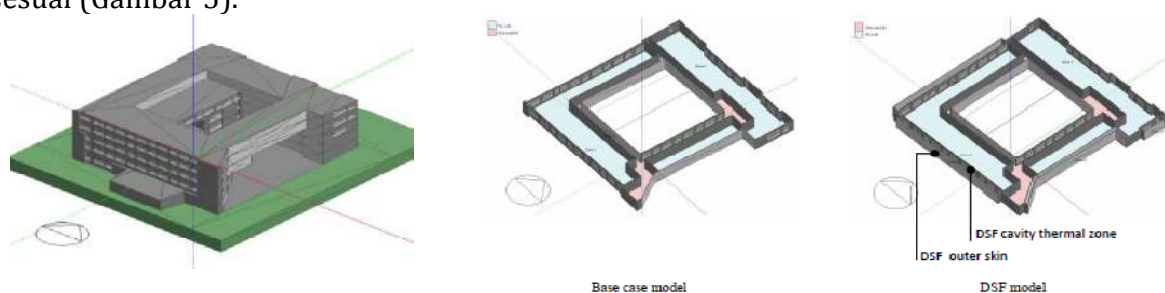
Gambar 5. Model Dasar dan Model DSF Pada Program Simulasi
